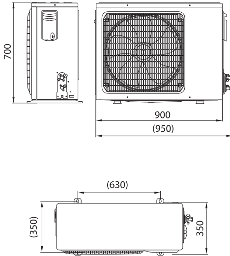
Размеры: BLCI_O/out-36HN8/EU BLCI_O/out42HN8/EU
