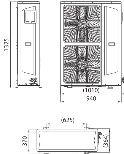
Размеры: BLCI_O/out-48HN8/EU BLCI_O/out-60HN8/EU
