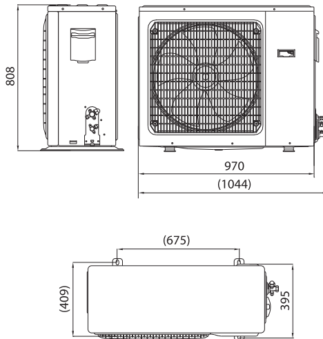
Размеры: BLCI_O/out-36HN8/EU BLCI_O/out42HN8/EU
